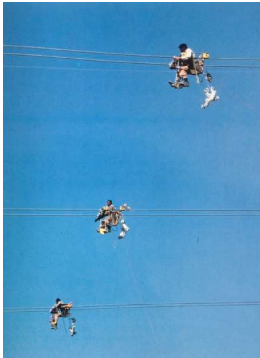
POSA DEI DISTANZIATORI
